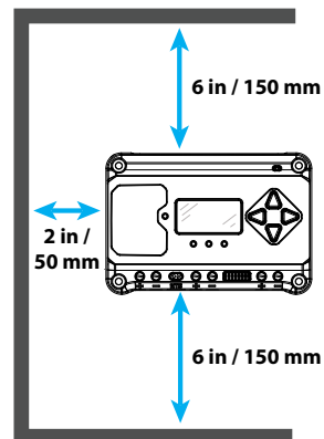
Abbildung 3.1 – Korrekte Abstände für passive Kühlung
